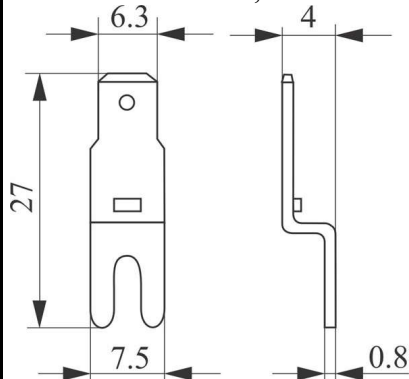
Kontakt za dizalice Kod 7108
