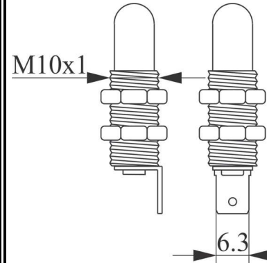
Kontakt zastavica za četkicu (grafitnu)
