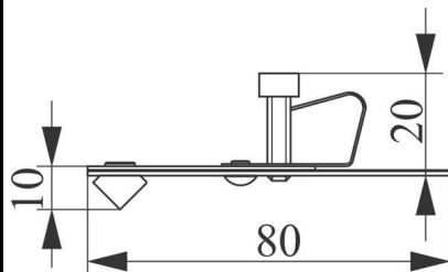
Držač kabla Kod 5611
