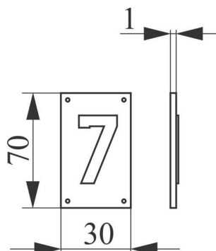
Aluminijumske cifre 0-9 Kod 5621
