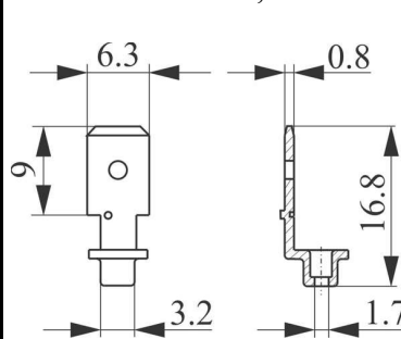
Kontakt zastavica za četkicu (grafitnu)
